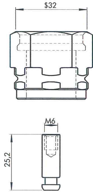
TA-R25
