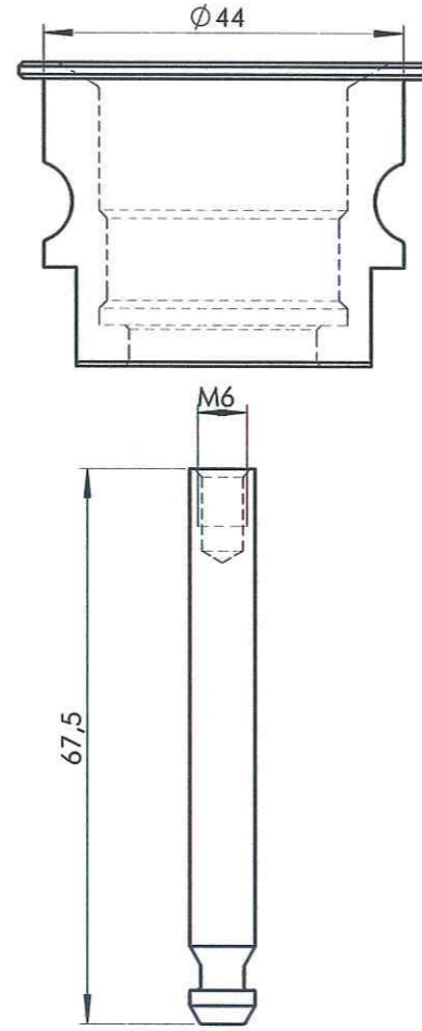
TA NV/NVG 24
