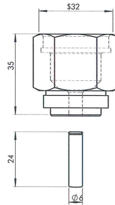
JCI VA-745x
