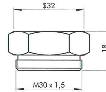
DANFOSS AMV 10,13,20,23
