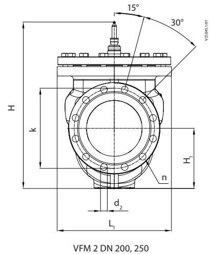
VFM 2 DN 200, 250
