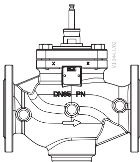
VFM 2 (DN 65-250)
